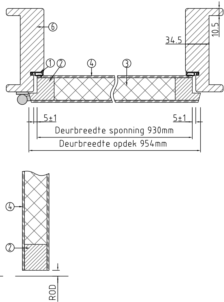
Doorsnede BB
