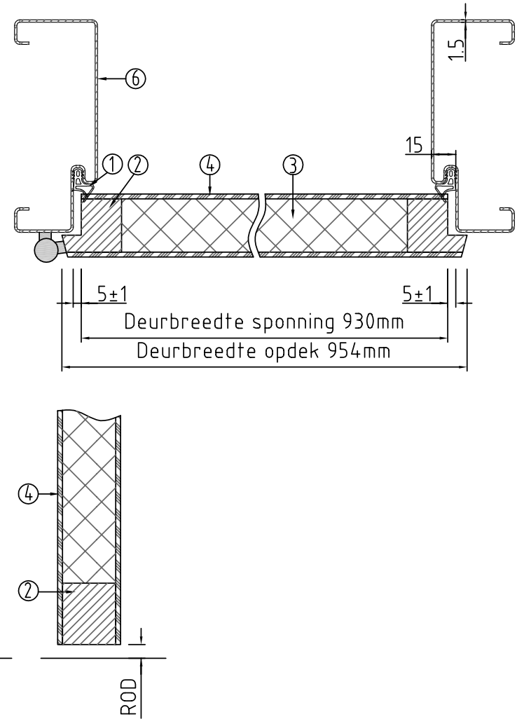
Doorsnede BB
