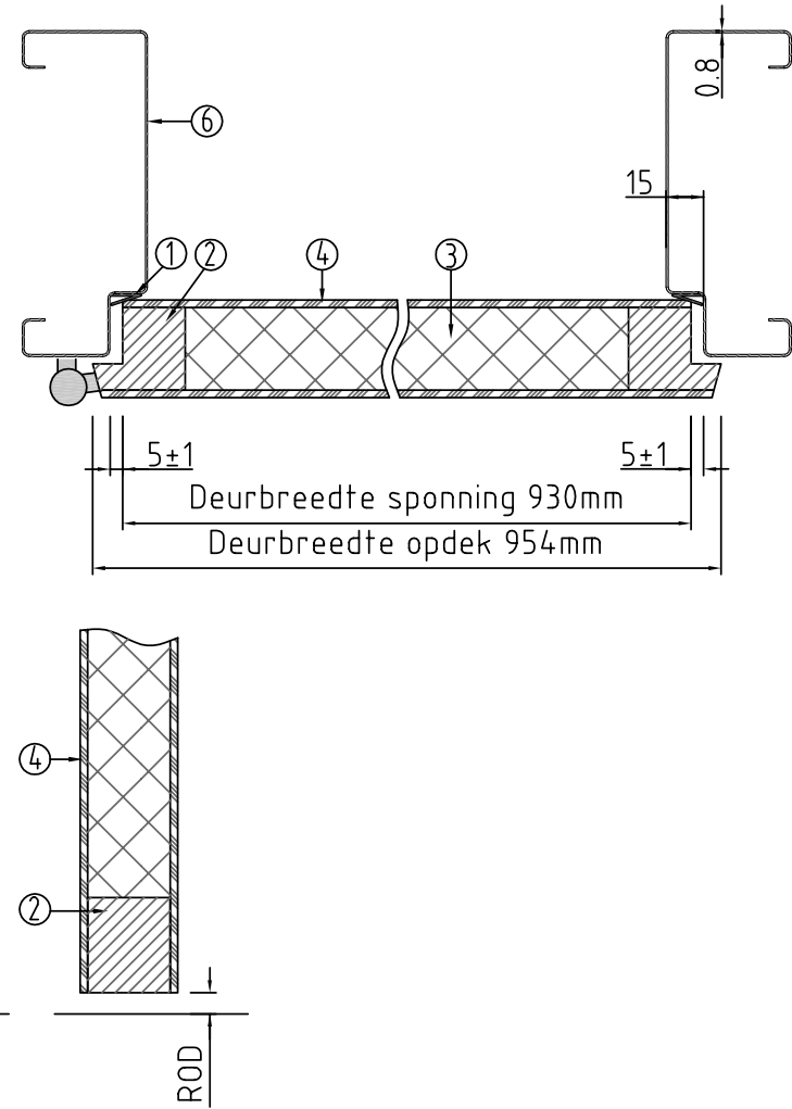
Doorsnede BB
