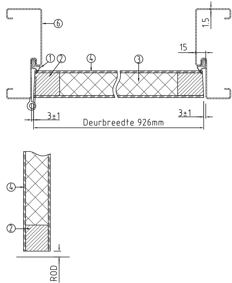
Doorsnede BB
