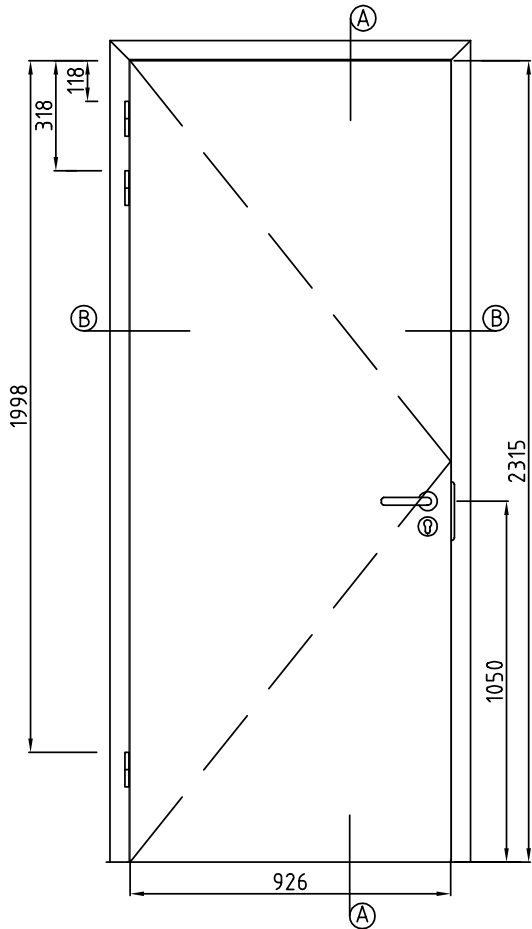
Vooraanzicht
