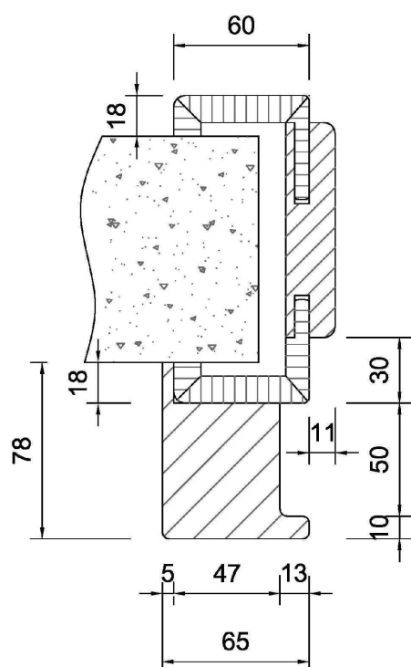
Aanslagkast + doorgangskozijn model 20, gemaatvoerd
