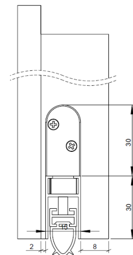
Valdorpel
