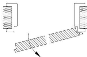
Rechtsdraaiende deur, constructieprincipe
