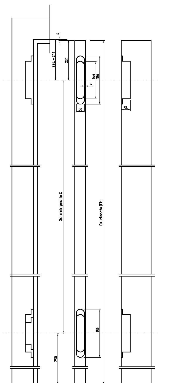
2 scharnieren
