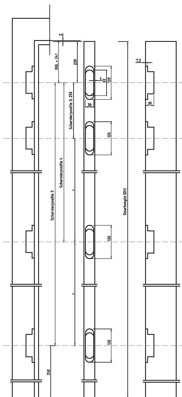
3 of 4 scharnieren
