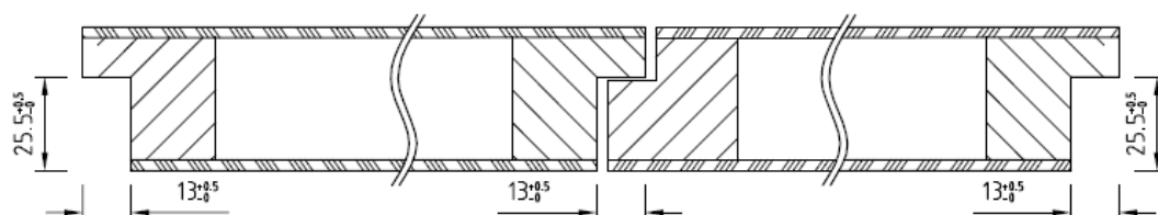
Opdek dubbeldeurs met tegensponning
