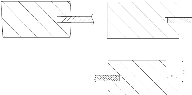
Profil (sans latte à vitrage)
