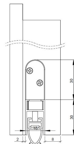
Plinthe automatique
