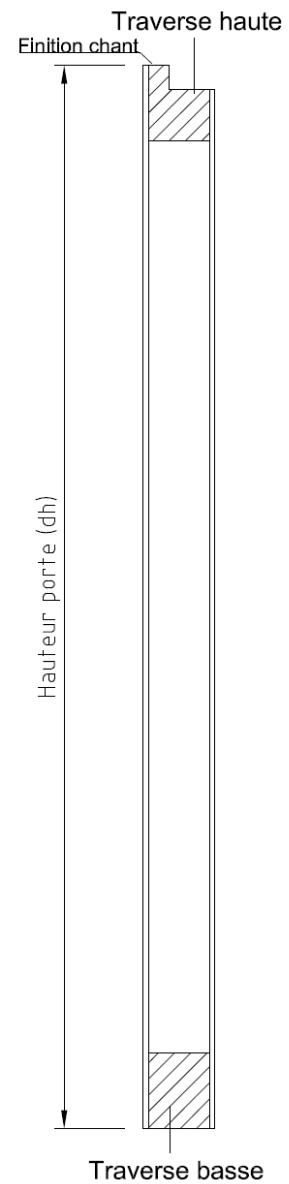
Coupe BB
