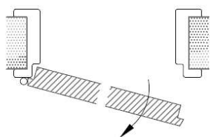
Porte gauche tirant Principe de construction
