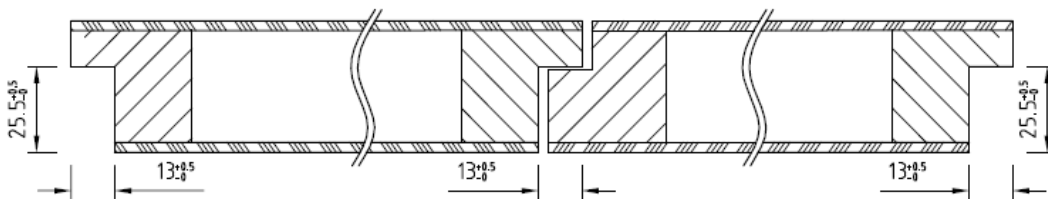
Vantail double à recouvrements , feuillure / contre feuillure
